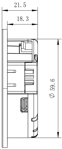
VUE LATÉRALE
