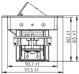
VUE LATÉRALE
