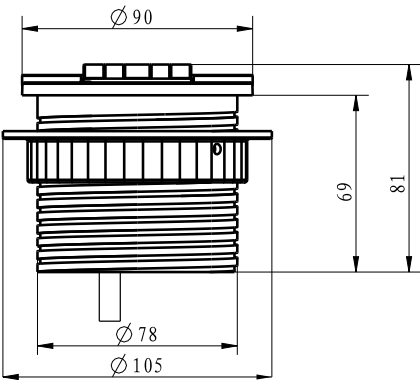
VUE LATÉRALE
