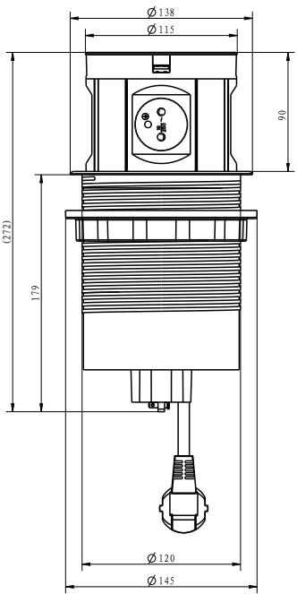
VUE DE FACE – OUVERT
