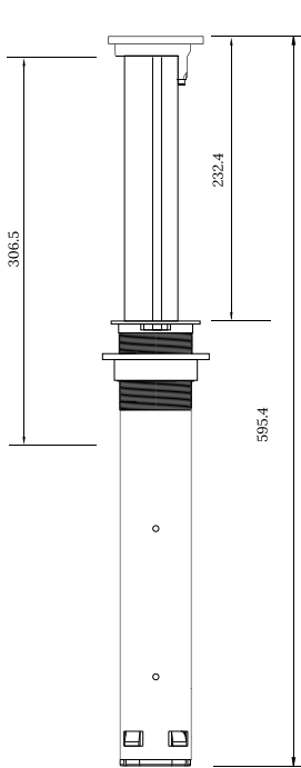
VUE DE FACE – OUVERT
